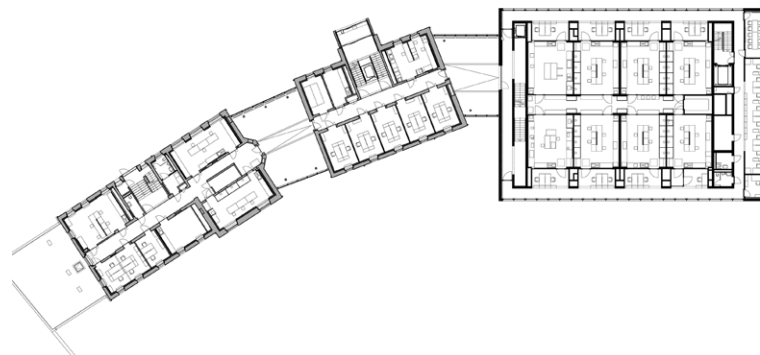
Plan du niveau 1
